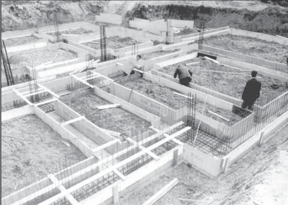
„Verlorene“ pecafil-Fundamentalschalung
