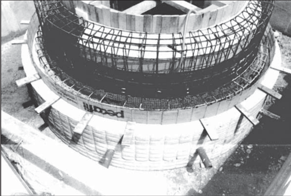
Rundschalungen aus pecafil-Universal-Schalmaterial VR6
