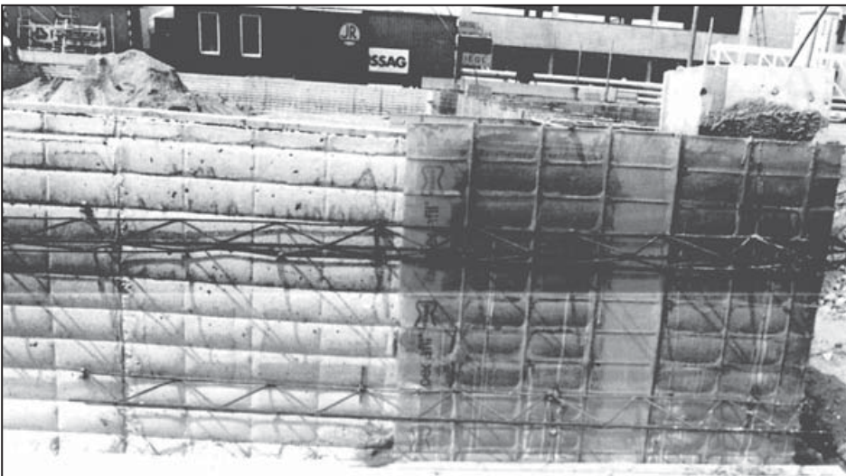
Wiedergewinnbare und mehrfach einsetzbare Fundamentalschalung
