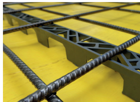
Zusätzliche Angaben zur Anordnung und zu den Verlegeabständen sind im DBV-Merkblatt enthalten.
